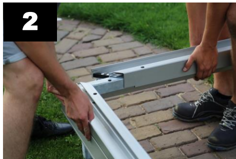
2 Schuif de hoekstukken in de liggers (4x).
